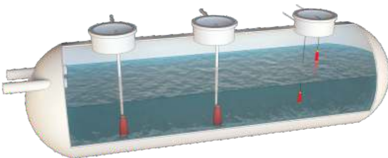
Tanque para tratamiento de aguas pluviales.
